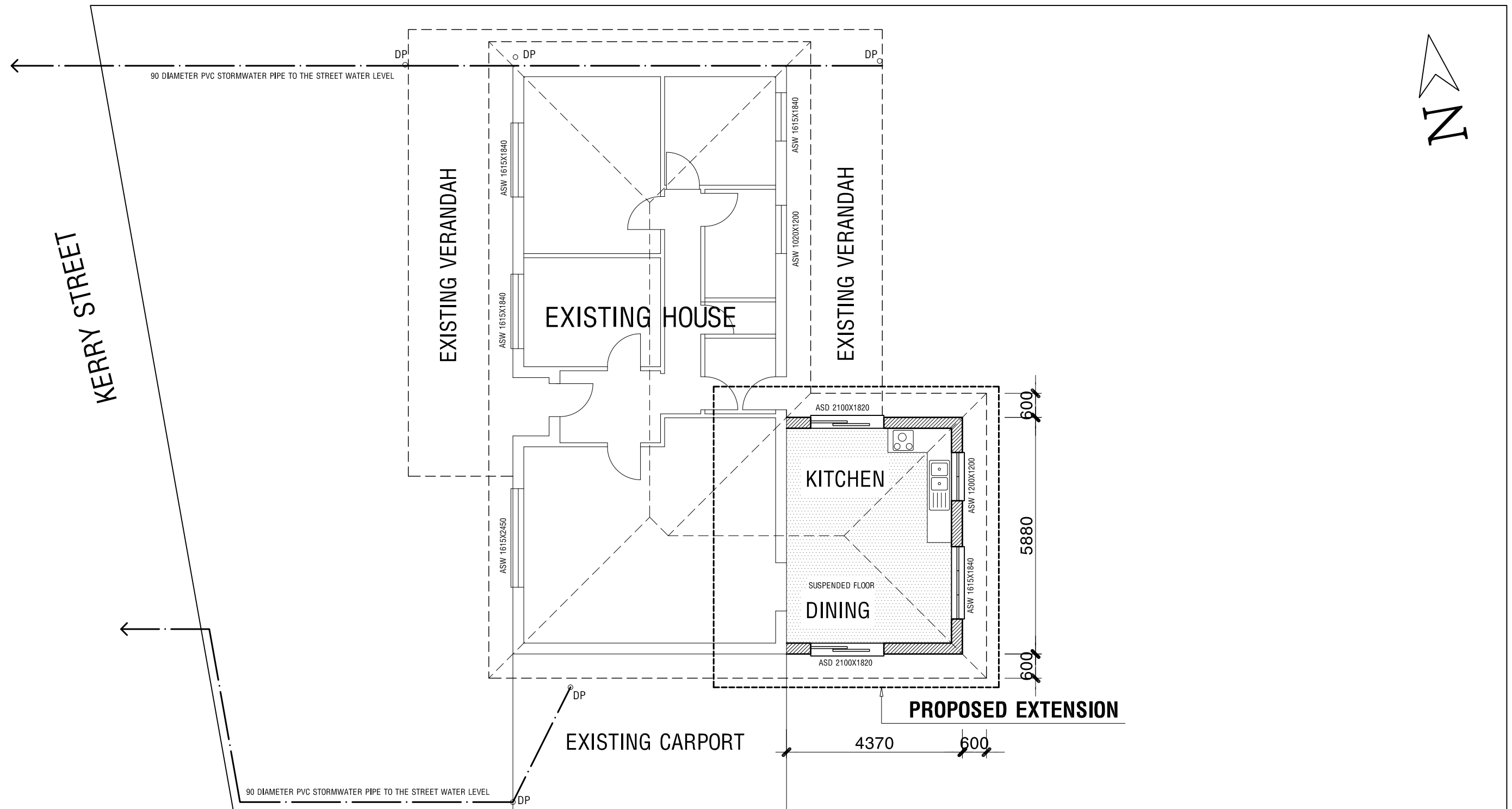
SITE PLAN 1:100
